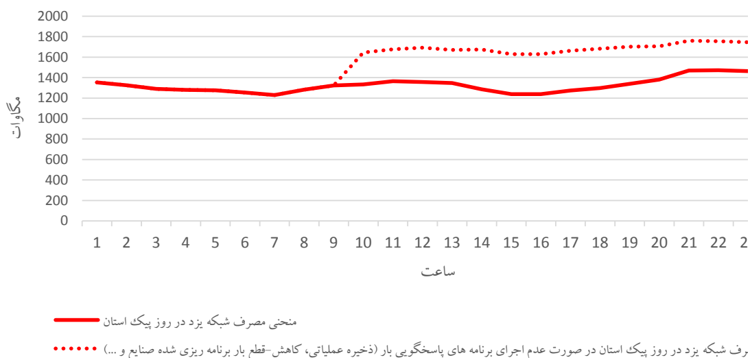
تأثیر همکاری صنایع در اجرای برنامه های پاسخگویی بار بر منحنی بار شبکه یزد در روز پیک استان (۱۴۰۱/۵/۴)
