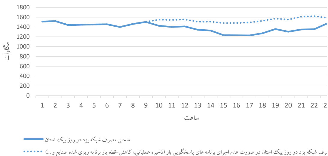
تأثیر همکاری صنایع در اجرای برنامه های پاسخگویی بار بر منحنی بار شبکه یزد در روز پیک سراسری کشور (۱۴۰۱/۵/۲۵)
